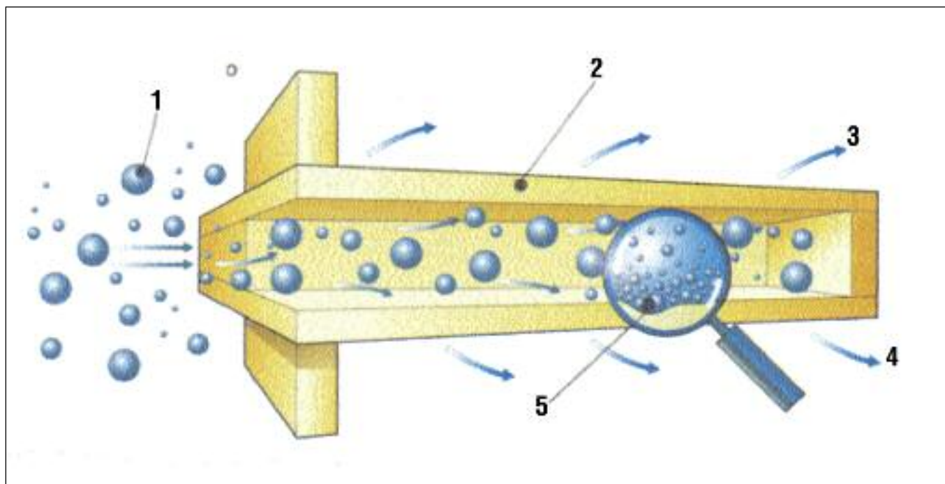
Diseño de los filtros FAP. constituidos por una cantidad de pequeños canales cerrados en los extremos. 1- Gases de escape con polvo. 2 Paredes porosas de un canal del filtro. 3- Gases de escape limpios. 4- Gases limpios. 5- Hollín en las paredes del canal.
